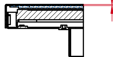
A-A (1:2)
